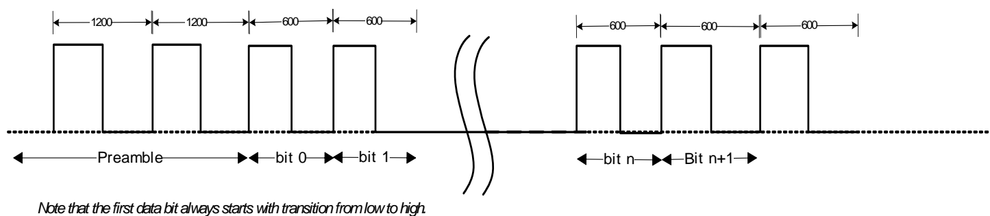
Figure 3 - OOK LF packet structure
